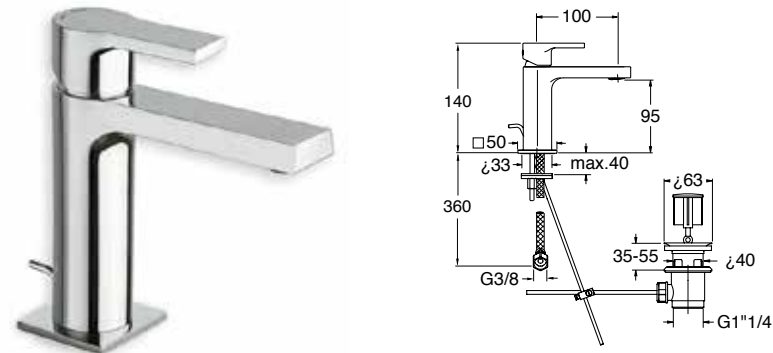
➤ Art. AB162 Miscelatore monocomando per lavabo con scarico da 1"1/4 e asta comando Single handle faucet for washbasin with 1"1/4
