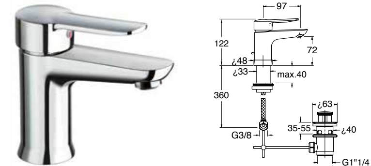
➤ Art. AB163 Miscelatore monocomando per lavabo con scarico da 1"1/4 e asta comando Single handle faucet for washbasin with 1"1/4
